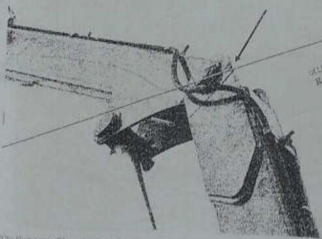
02-Fotografia de detalhe, onde indicam-se os vestígios de fundimento térmico elétrico na região de contato entre o guincho e a rede de energia elétrica.
